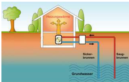
PdC acqua-acqua
