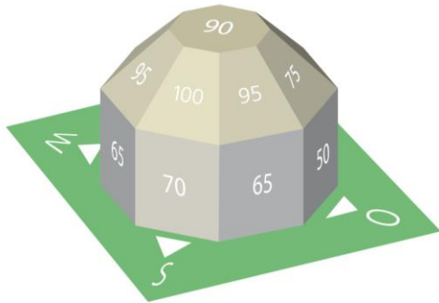
Percentuale di irraggiamento solare su superfici con vari orientamenti ed inclinazioni, rispetto al massimo (sud, 30° di inclinazione), riferito all'altopiano svizzero.
